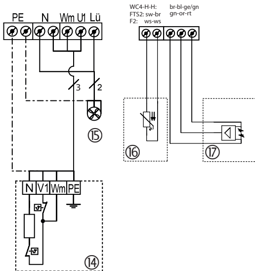
Afb. 6: Aansluitschema uitbreidingsplatine
