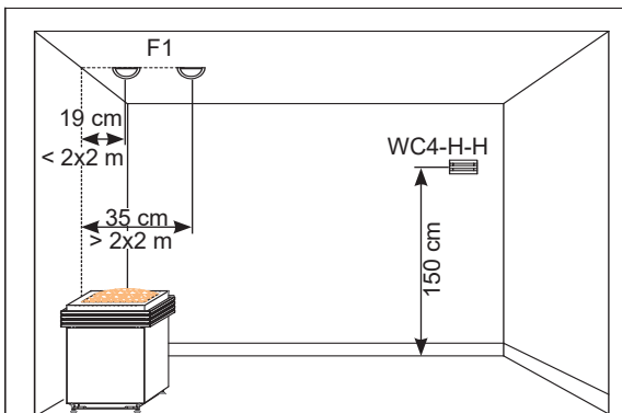
Abb. 3: Montage Fühler
