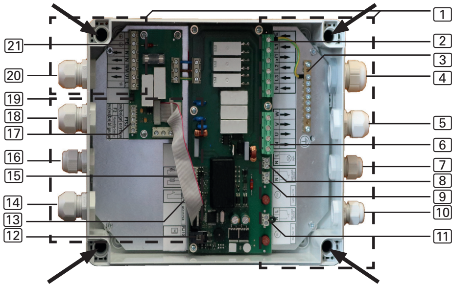
Afb. 4: Elektrische aansluiting
