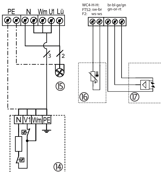
Abb. 6: Anschlussplan Erweiterungsplatine
