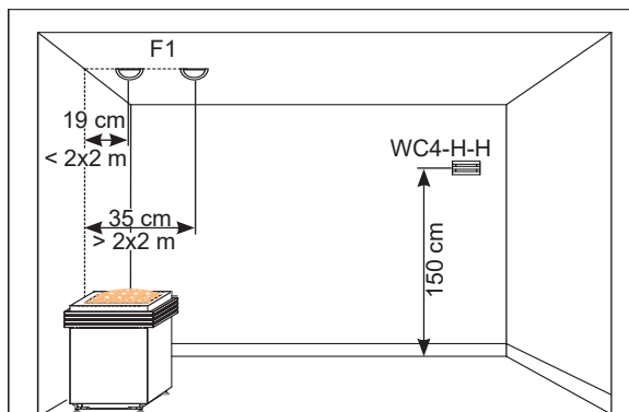
Bild 3: Montering givare
