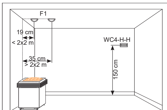
Afb. 3: Montage voeler
