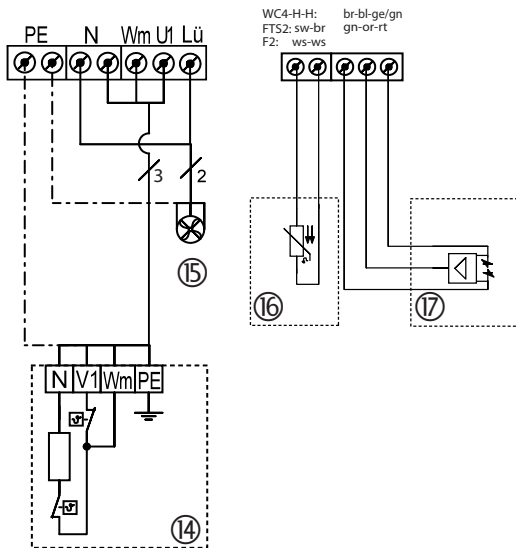
Kuva. 6: Liitântäkaavio – laajennuspiirilevy
